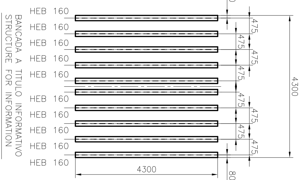
BANCADA A TITULO INFORMATIVO STRUCTURE FOR INFORMATION
